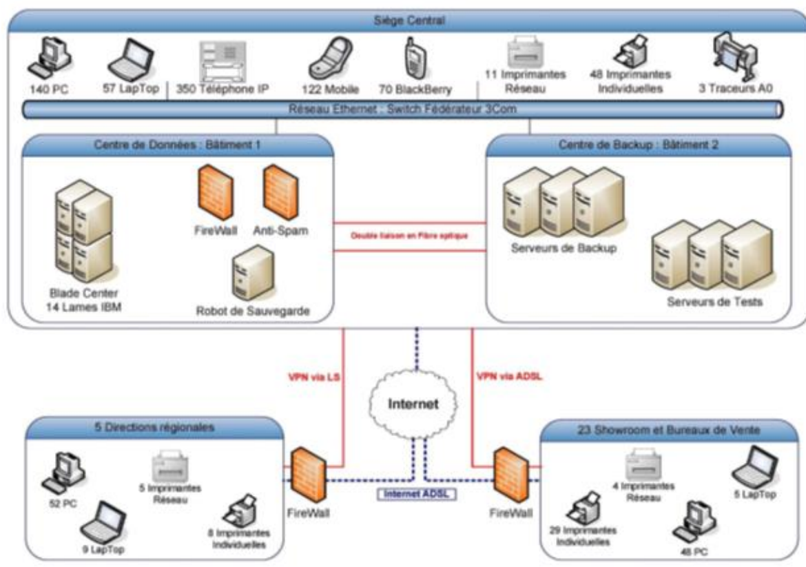
Figure 33 Schéma de l'architecture réseau du système d'information
