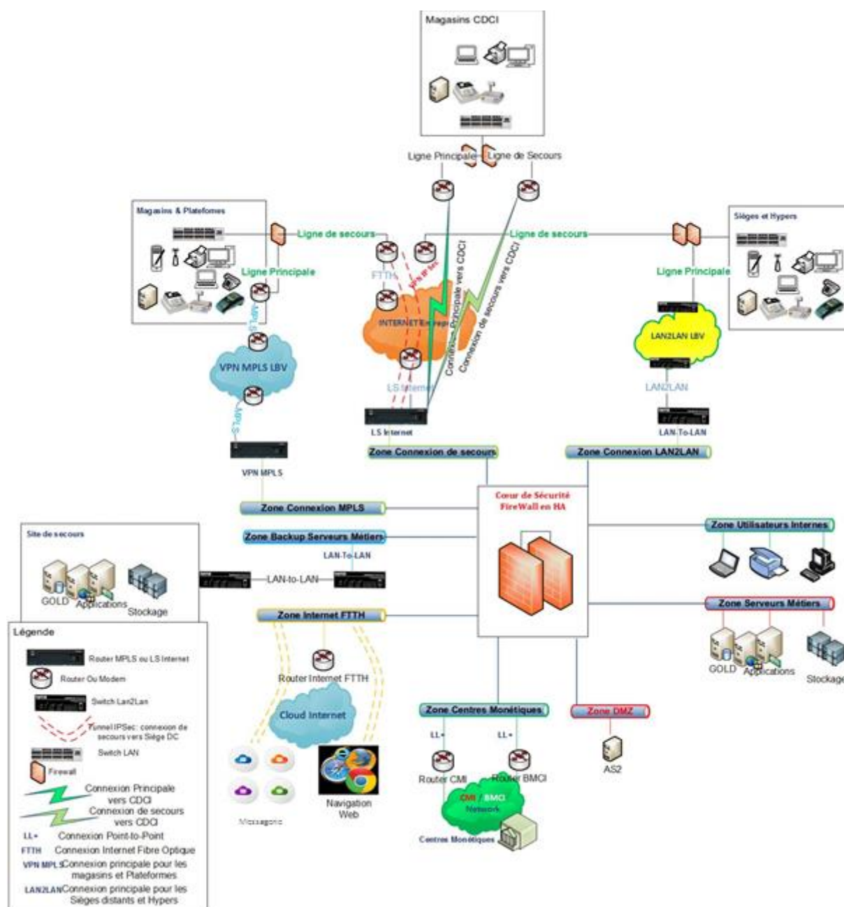
Figure 29 : L'architecture du Système d'Information
